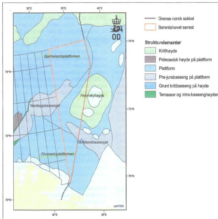
Figur 5.1 Oversikt over geologiske strukturelementer i sørøstlige del av Barentshavet.
